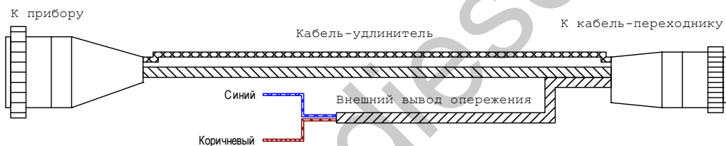
Рисунок 21. Кабель-удлинитель
