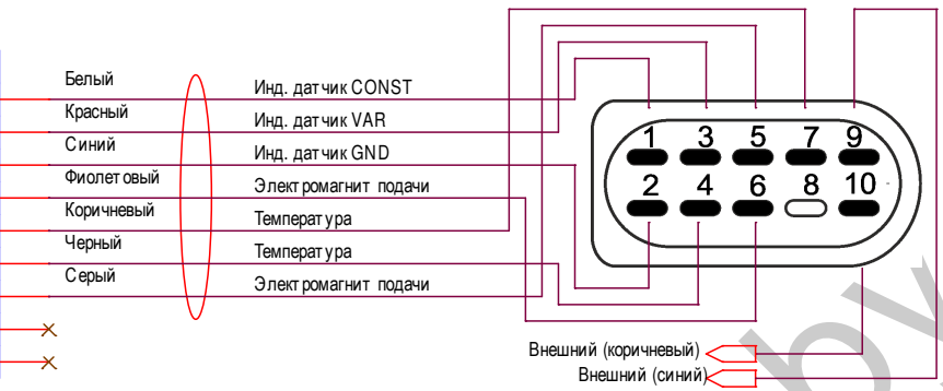
Рисунок 17. Разъем ТНВД тип 4
