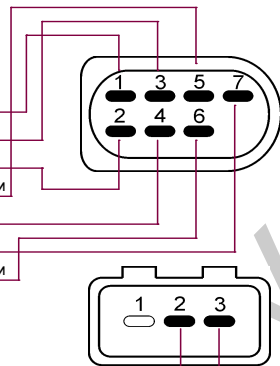
Рисунок 11. Схема распайки разъема ТНВД тип 1
