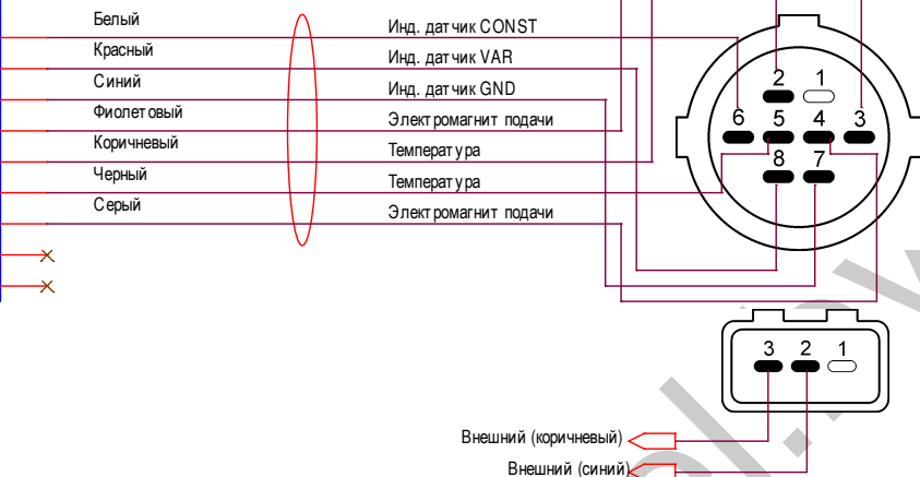
Рисунок 13. Схема распиновки разъема THVD тип 2
