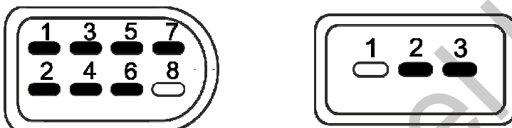
Рисунок 18. Разъем ТНВД тип 5: а – подача и индуктивный датчик, б – клапан опережения
