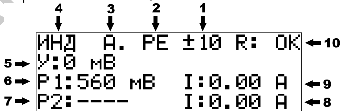
Рисунок 5. Описание информации на индикаторе прибора режим PE
