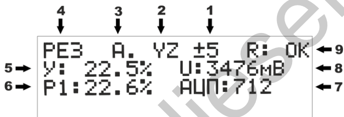
Рисунок 6. Описание информации на индикаторе прибора режим YZ
