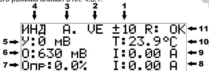
Рисунок 4. Описание информации на индикаторе прибора режим VE
