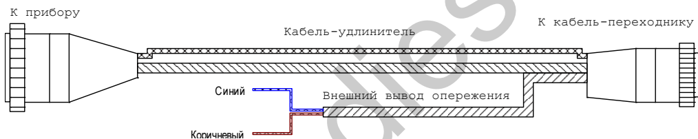
Рисунок 18. Кабель-удлинитель
