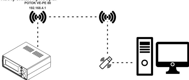
Рисунок 15. Подключение компьютера к прибору через USB адаптер
